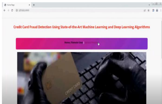
Fig.2. Login page.
